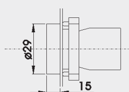
RP2-BA8+RP2-BZ10=RCP2-BA8
