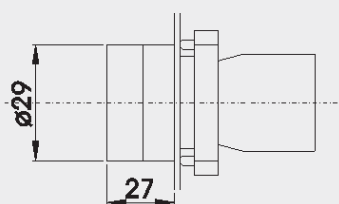
RP2-BD2+RP2-BZ10=RCP2-BD2 RP2-BD3+RP2-BZ10=RCP2-BD3
