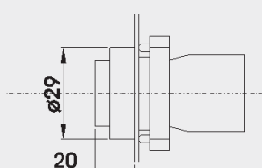
RP2-BL+RP2-BZ10=RCP2-BL
